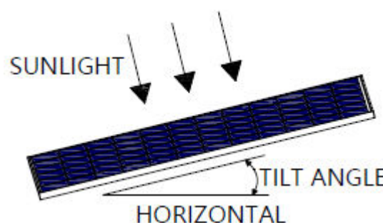
Figure1: PV module tilt angle
